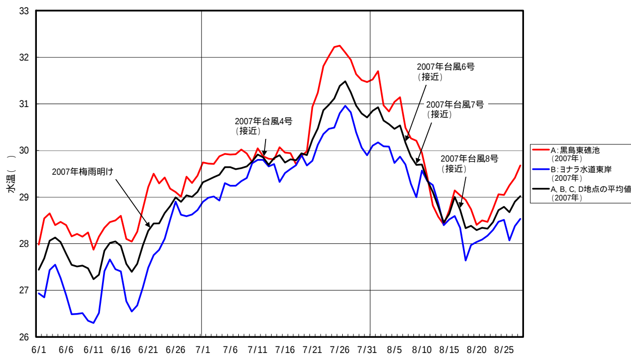
2007 年の日平均水温の地点間比較
