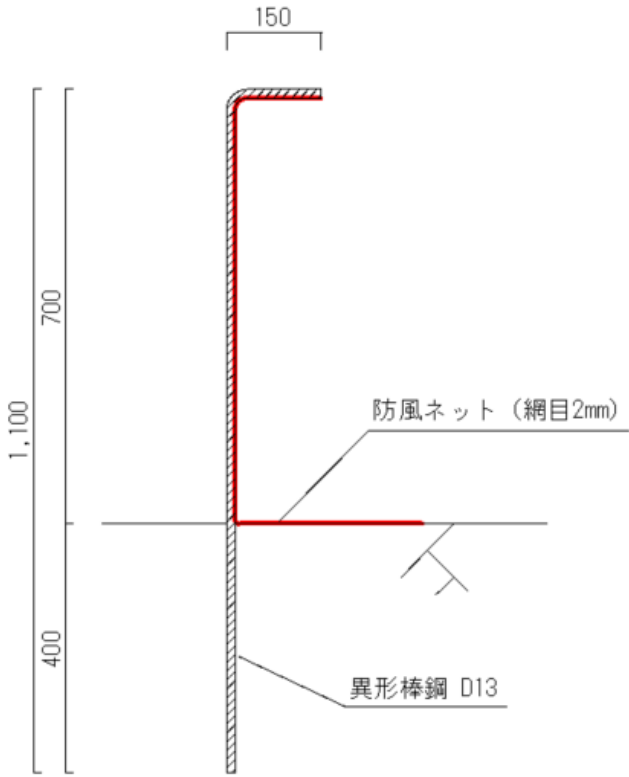
構造図
