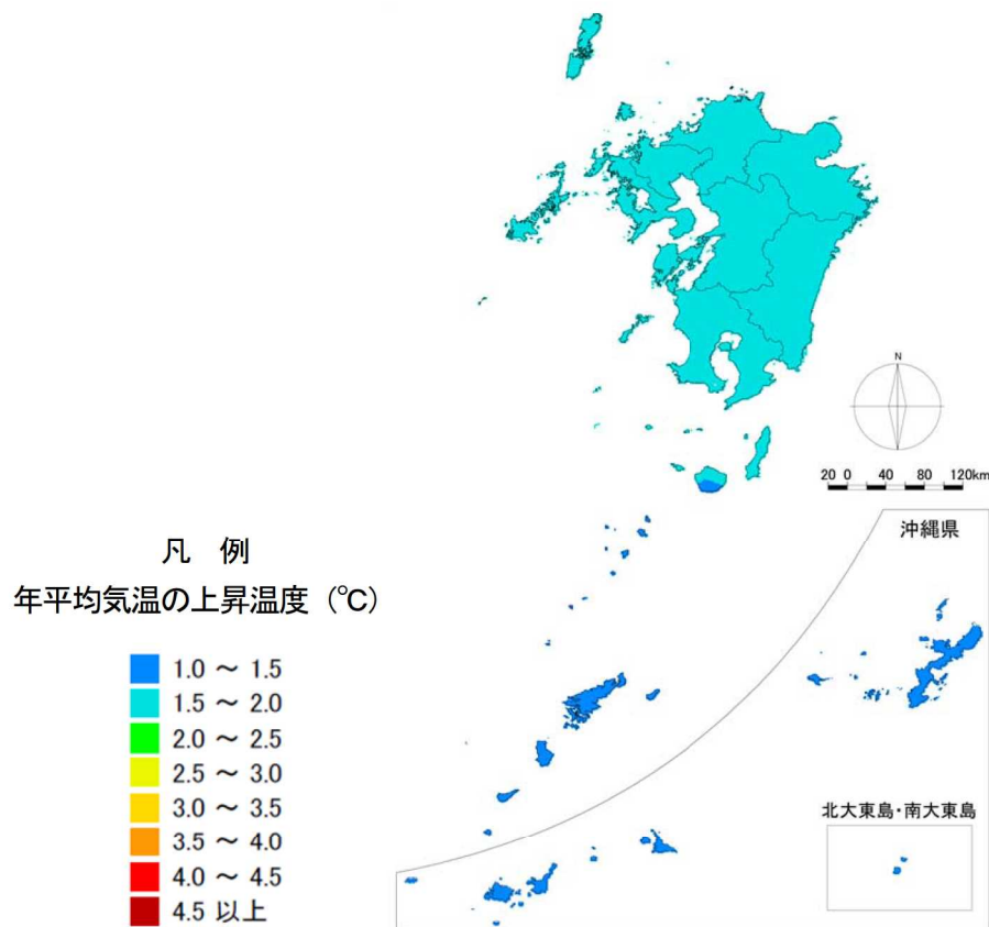
図 20 21 世紀末における九州・沖縄地方の年平均気温の上昇温度の予測 RCP2.6 MIROC5
