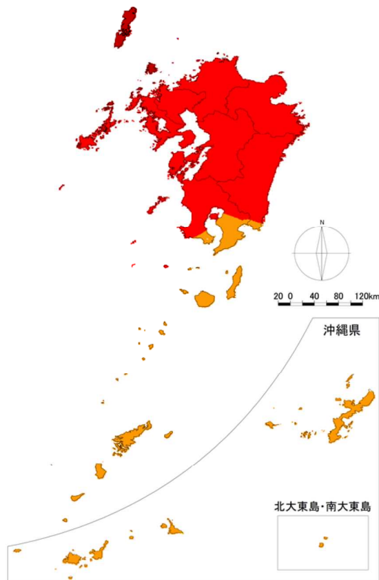
図 19 21 世紀末における九州・沖縄地方の年平均気温の上昇温度の予測 RCP8.5 MIROC5
