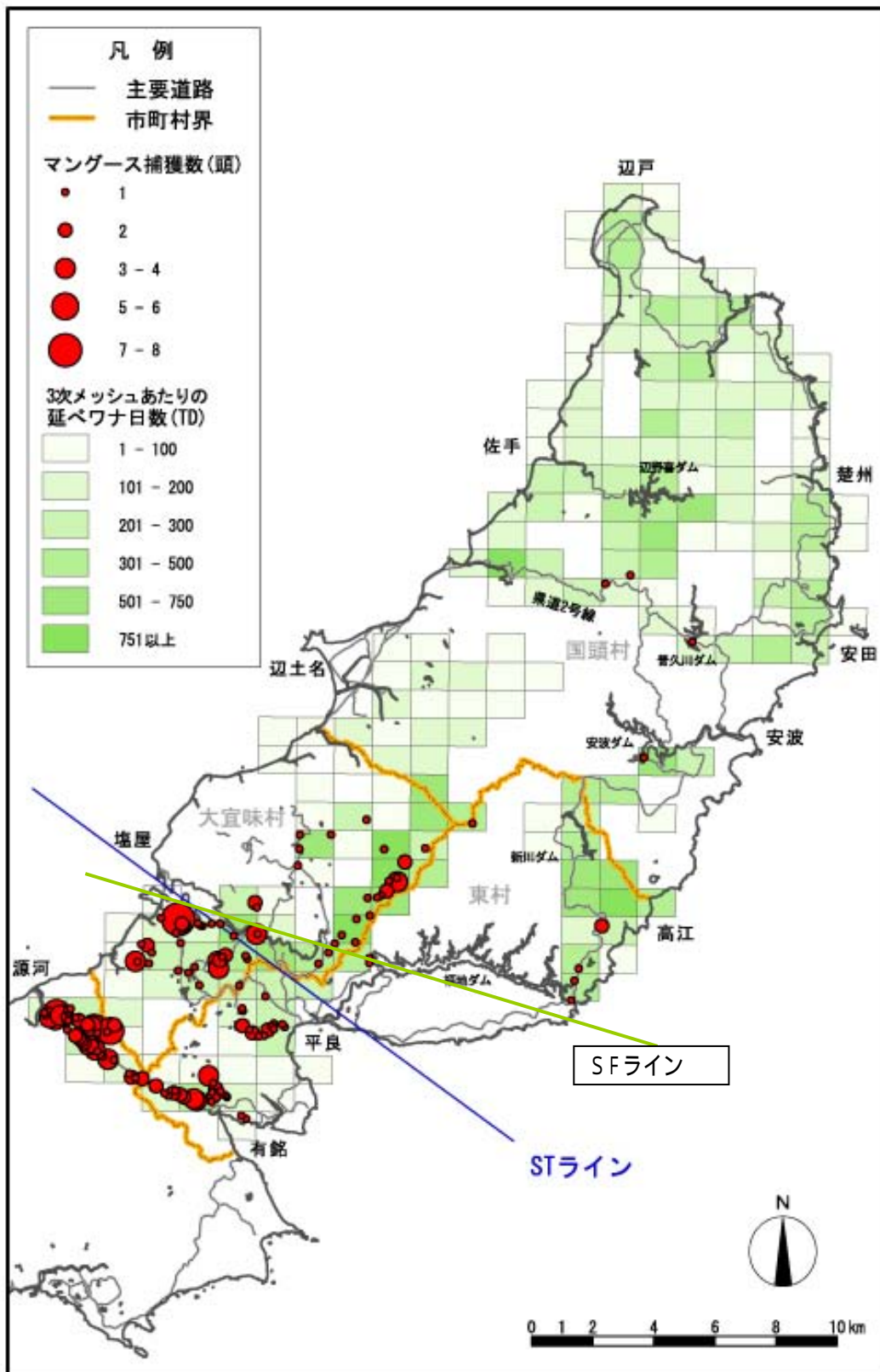
図2 平成17年度環境省マンゲース捕獲状況(4月～3月)
